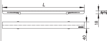
Abdeckung CeraLine Standard, verriegelbar
