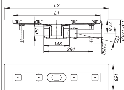
Duschrinne CeraLine F 500 – 1200
