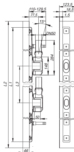
Duschrinne CeraLine W Duo 1100 – 2000
