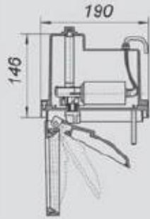
Çekvalf F tipine dönüştürme modülü stausafe F conversion module
