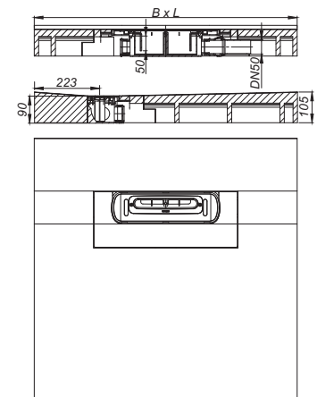
Duschelement DallFlex Floor
