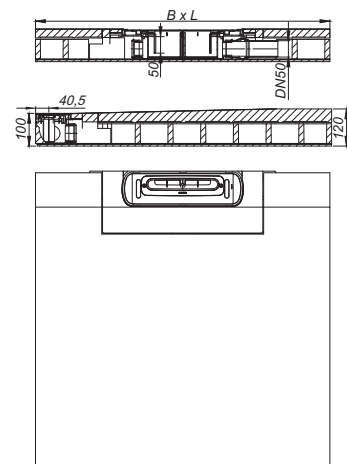
Schallschutz-Duschelement DallFlex Wall
