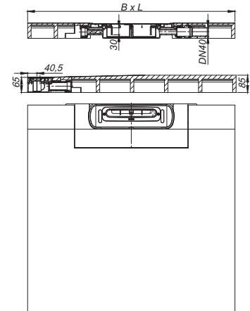
Duschelement DallFlex Wall Plan
