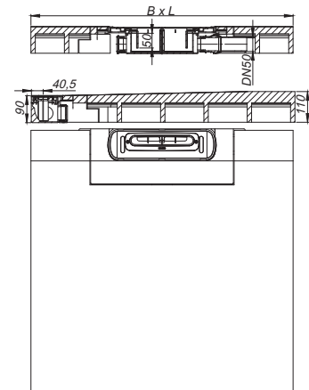
Duschelement DallFlex Wall
