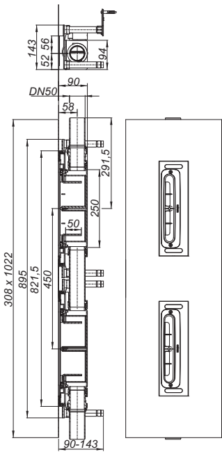
Ablaufgehäuse DallFlex Duo
