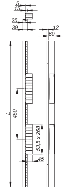
Duschrinne CeraWall Select N Duo Edelstahl matt
