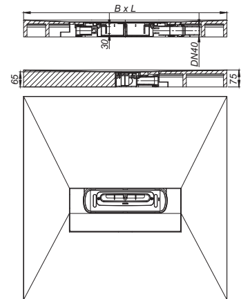
Duschelement DallFlex Compact Plan
