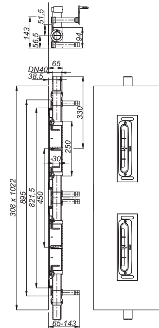
Ablaufgehäuse DallFlex Duo Plan
