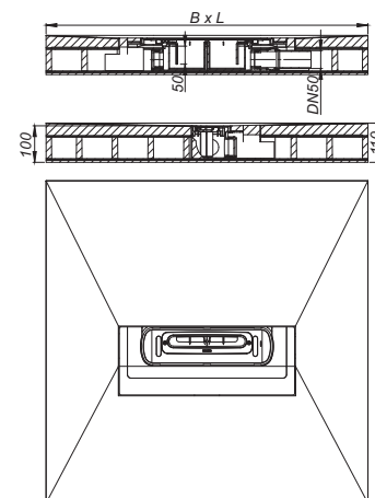
Schallschutz-Duschelement DallFlex Compact
