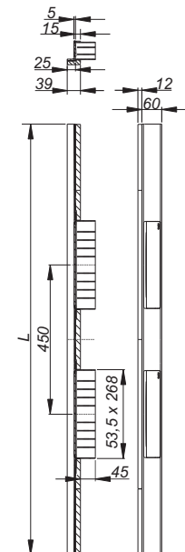
Duschrinne CeraWall Select N Duo Edelstahl poliert
