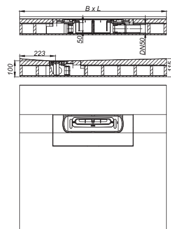
Schallschutz-Duschelement DallFlex Floor
