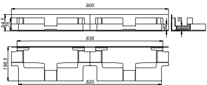
Schallschutzelement DallFlex Duo
