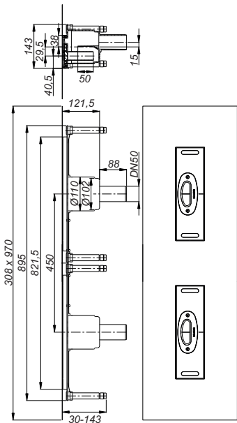
Ablaufgehäuse DallFlex Duo senkrecht
